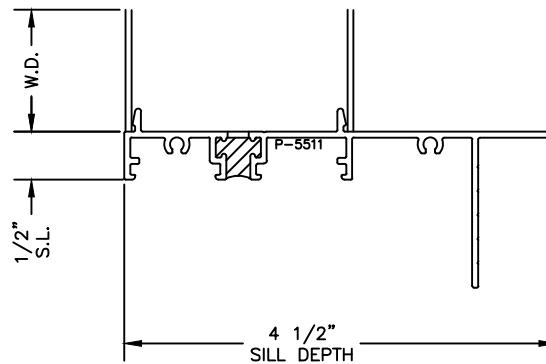
NAIL FIN ADAPTOR
