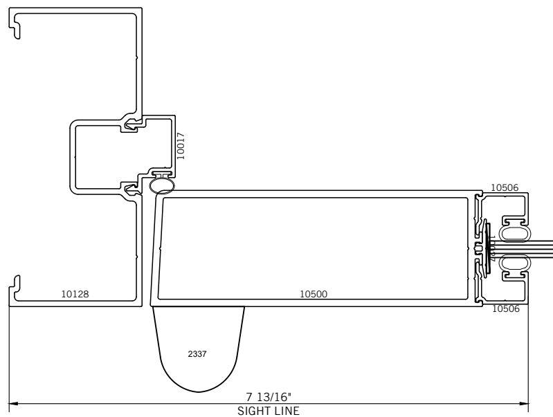
OFFSET PIVOT
