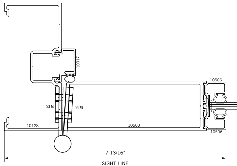
BUTT HINGE
