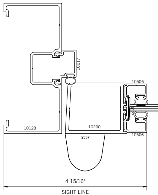
OFFSET PIVOT
