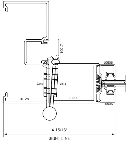
BUTT HINGE
