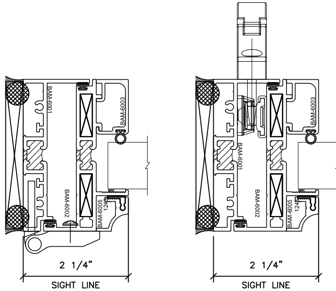
BUTT HINGE
