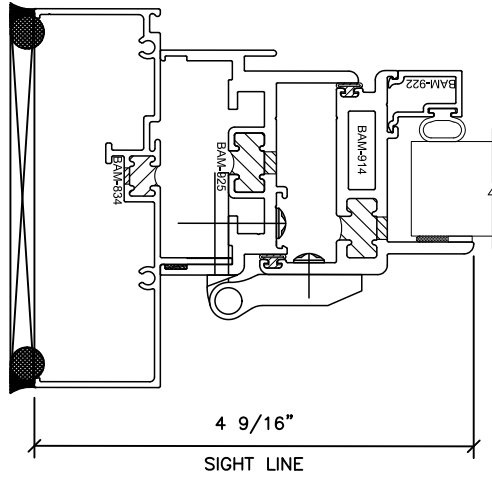
BUTT HINGE
