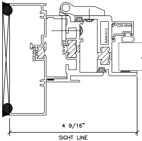
BUTT HINGE
