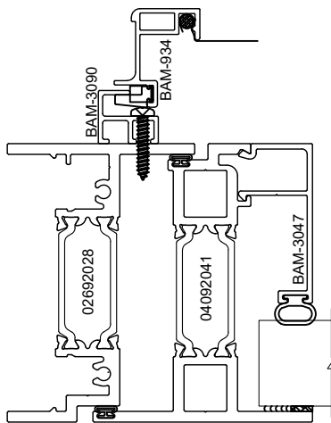
JAMB
