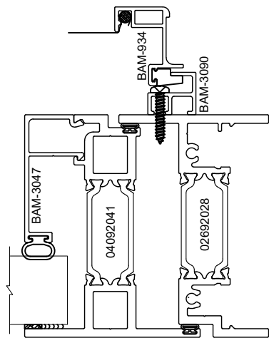
JAMB
