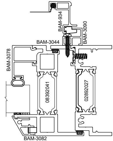
JAMB
