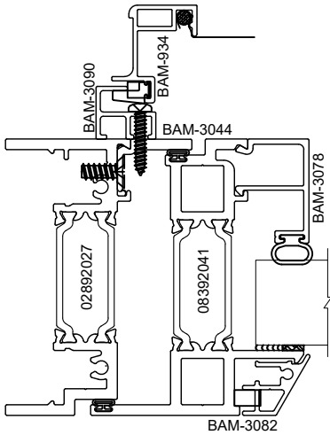
JAMB
