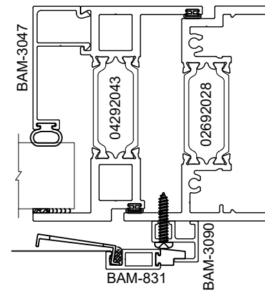
JAMB
