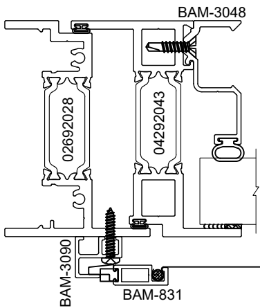
JAMB
