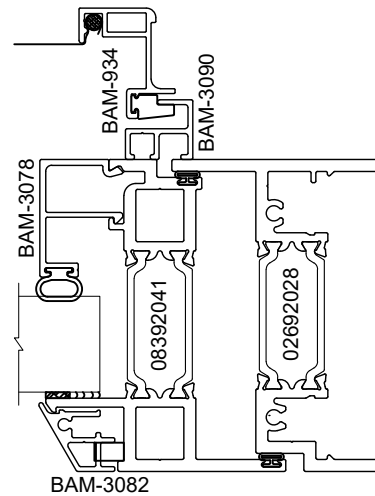
JAMB
