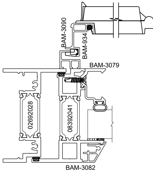
JAMB
