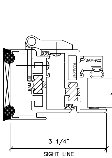
BUTT HINGE
