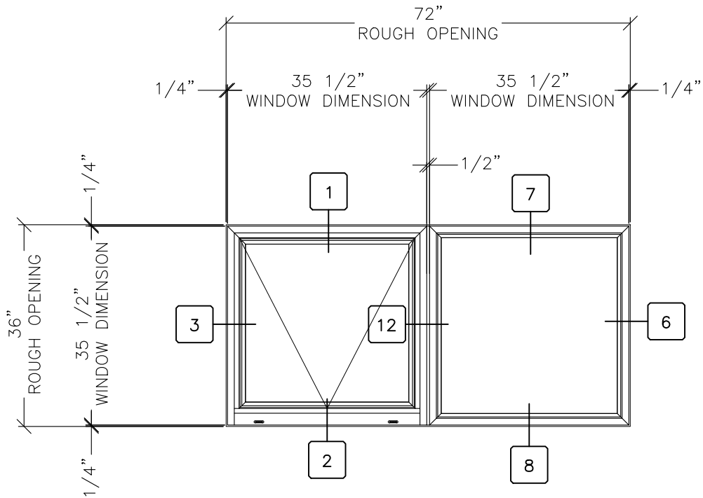
PROJECT IN /FIXED 522 MULLION
